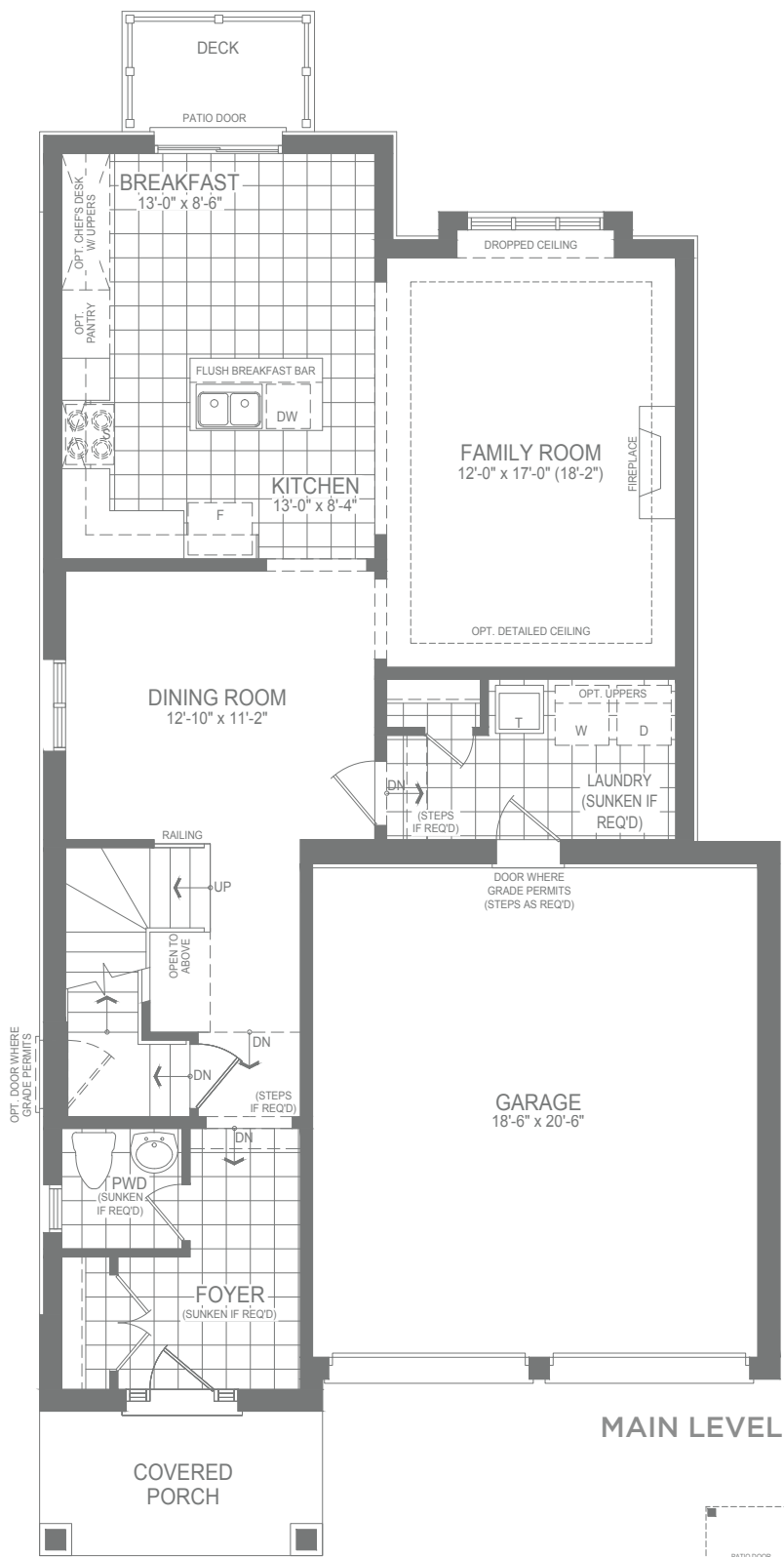
ELEV. C
