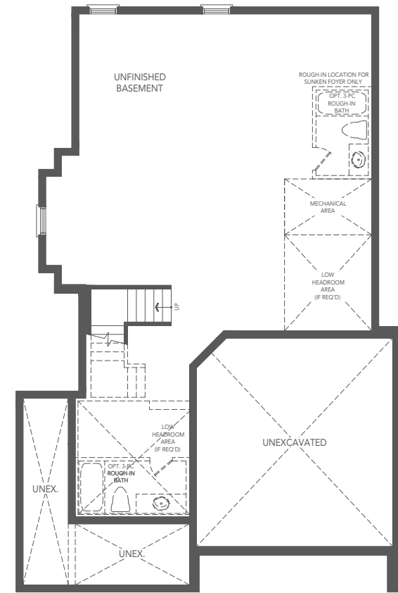
ELEV. B
