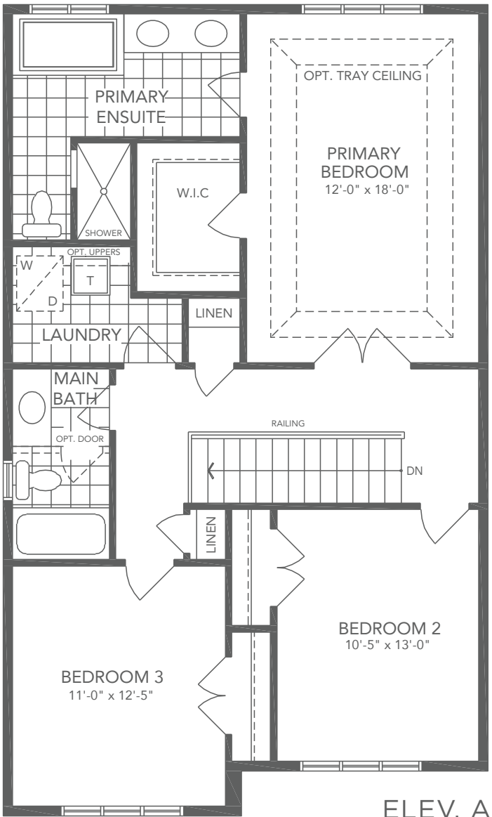
ELEV. A
