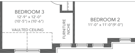
ELEV. D
